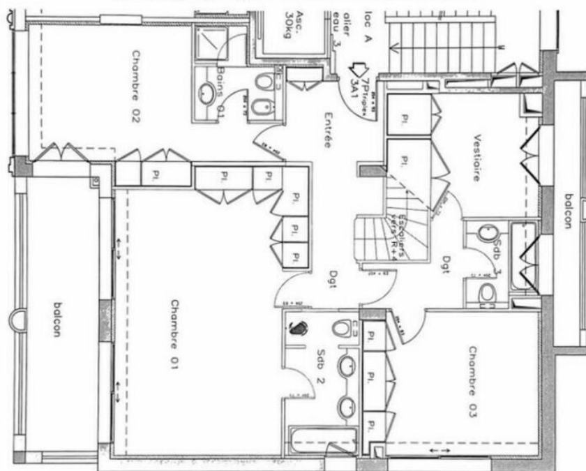
Plan modificatif - Appartements 3A1 + 4A1 - Niveau R+3
